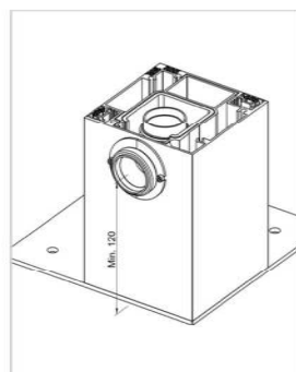
Corte Escoamento oculto L60/L70
